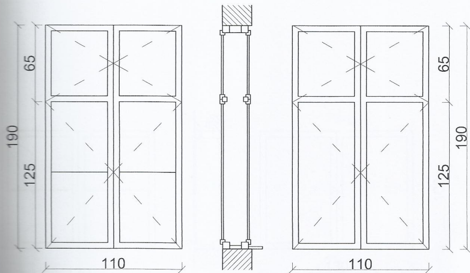
spoljašnji izgled
