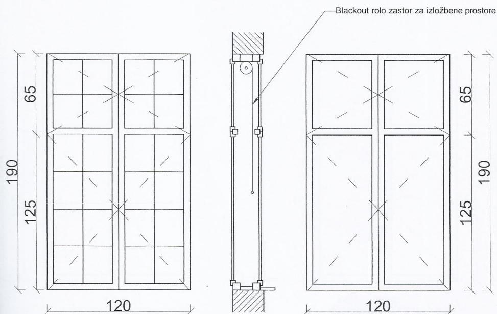
spoljašnji izgled
