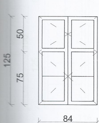
spoljašnji izgled
