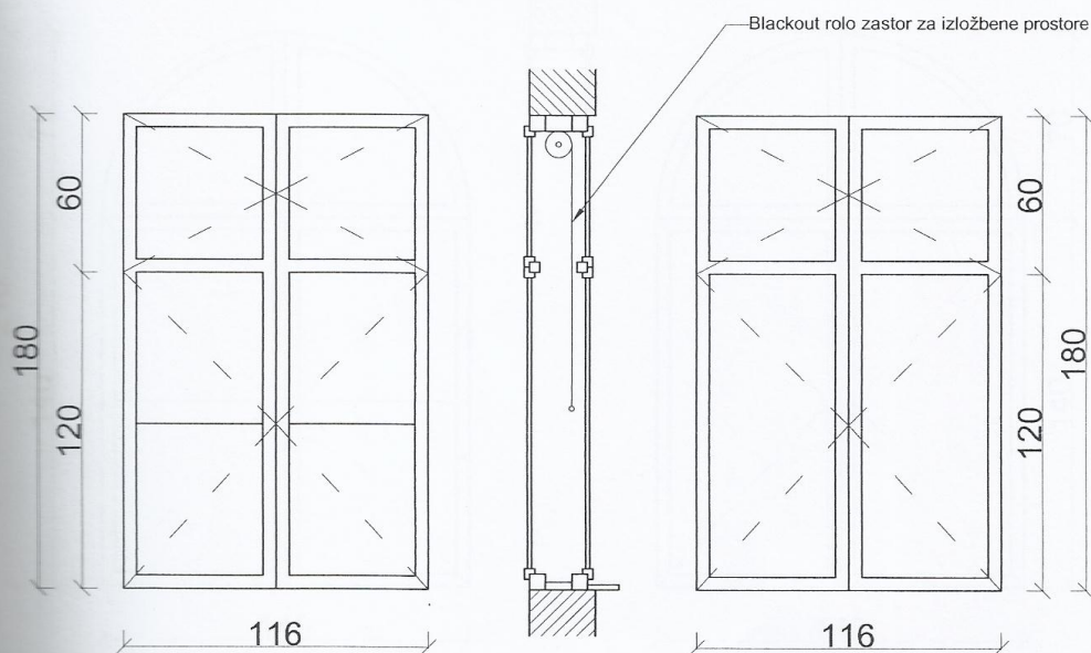
spoljašnji izgled
