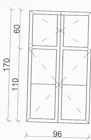
spoljašnji izgled
