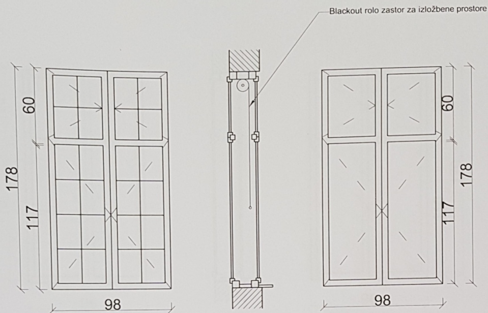
unutrašnji izgled
