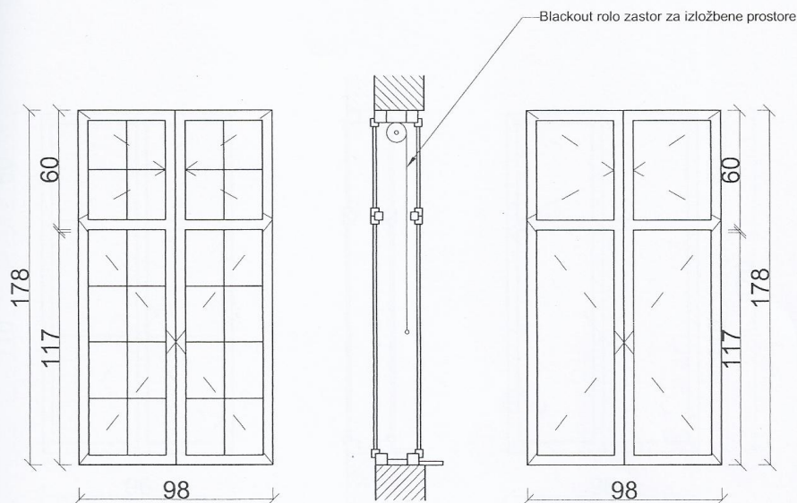
spoljašnji izgled
