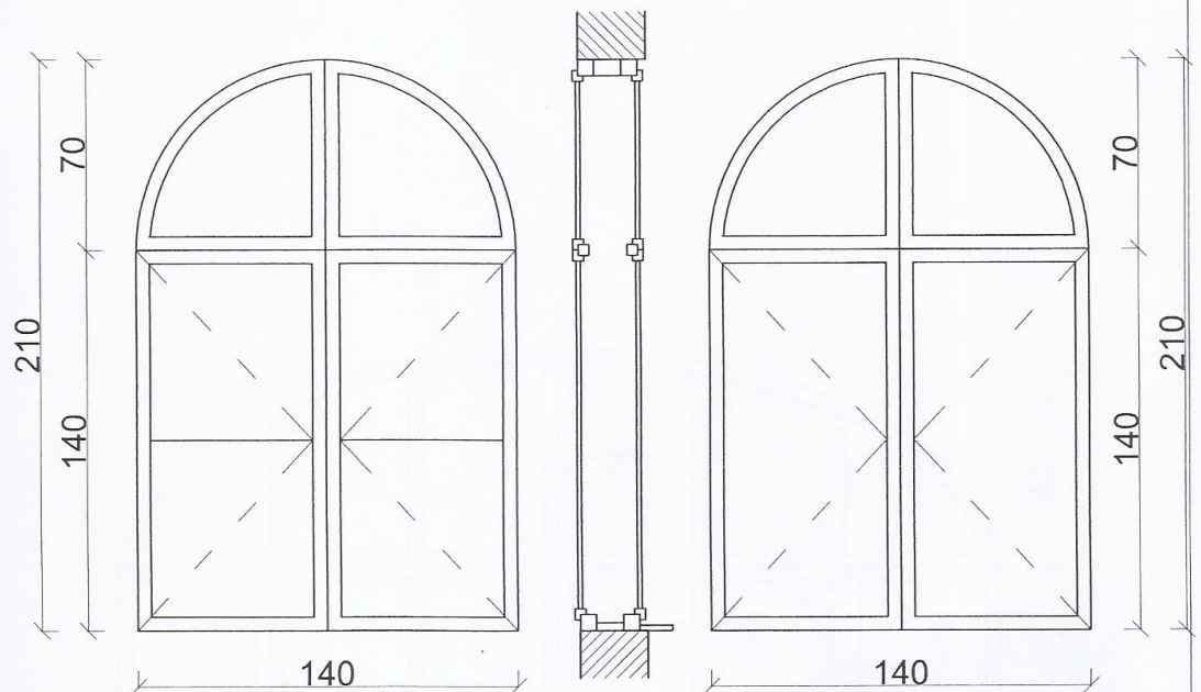
spoljašnji izgled
